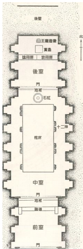
王建墓永陵墓室平面图 (图片来源：Wikimedia Commons)
