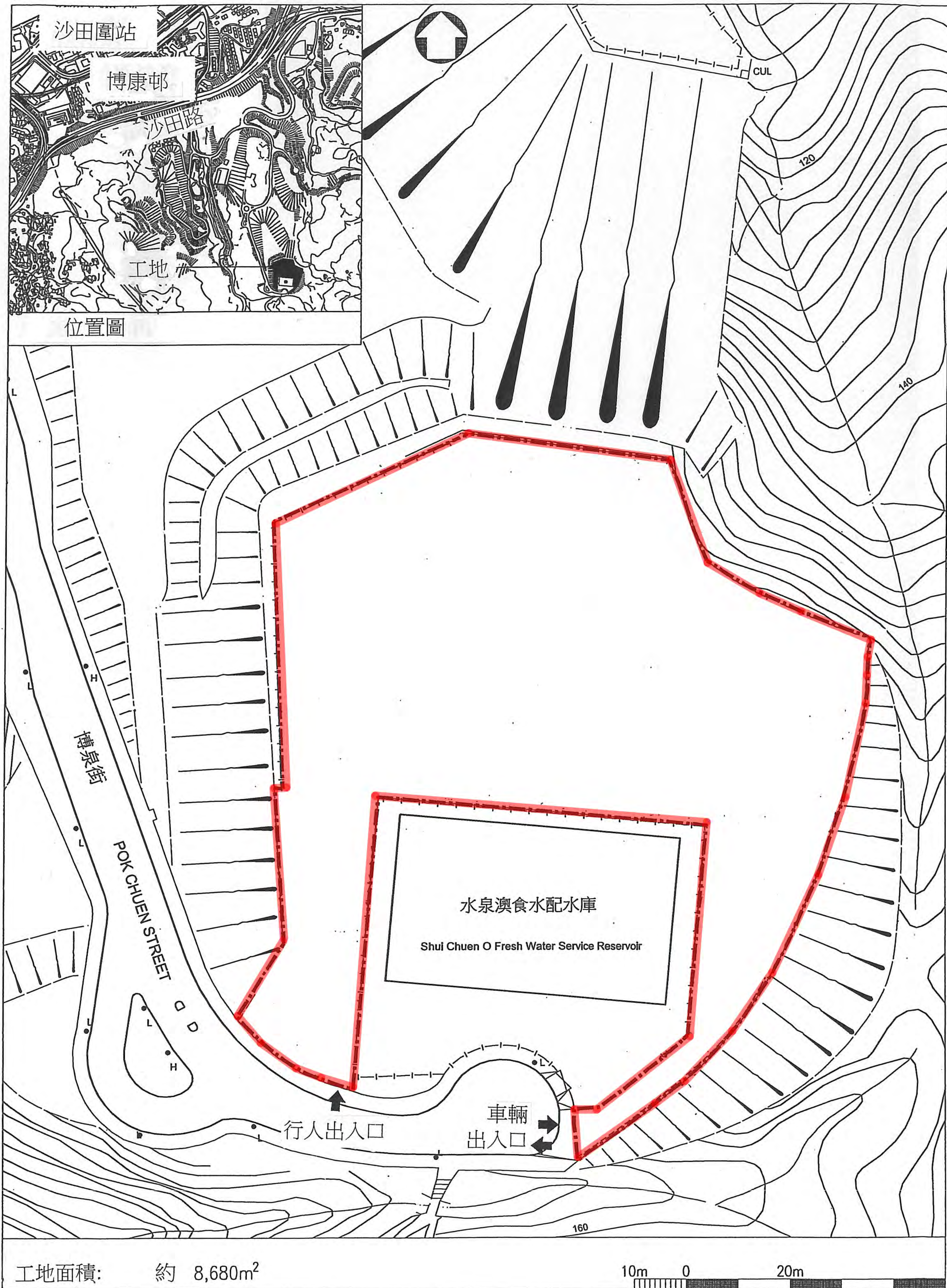
工地平面图 - 沙田水泉澳1所设有30间课室的小学
