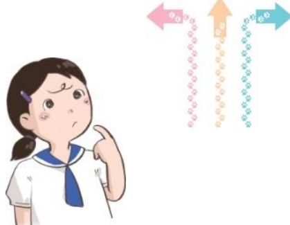
迷路
